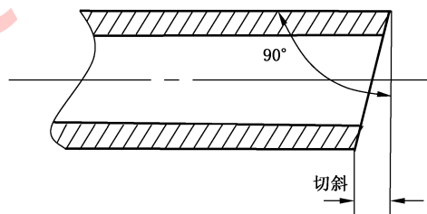
图 1 切斜
