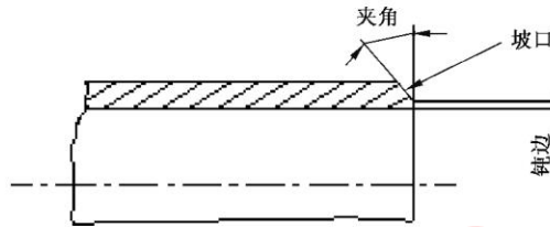
图 2 坡口示意图
